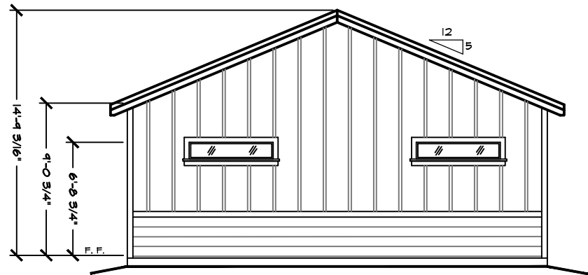
RIGHT ELEVATION
